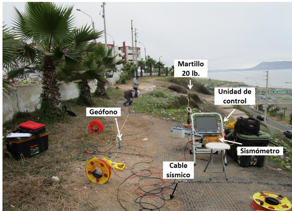
Figura 8. Equipos utilizados en la toma de datos según las técnicas SRT y MASW.
